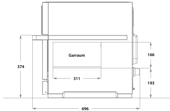
Seitenansicht
