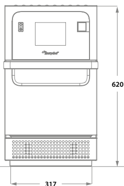
Frontansicht
