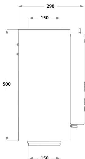
Seitenansicht
