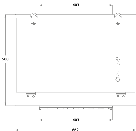
Frontansicht
